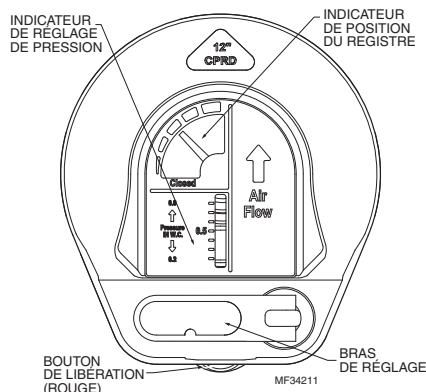
Fig. 4. Régulateur CPRD
